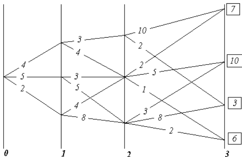
Рис. 1. К существованию метода динамического программирования. Матрица возможностей.
