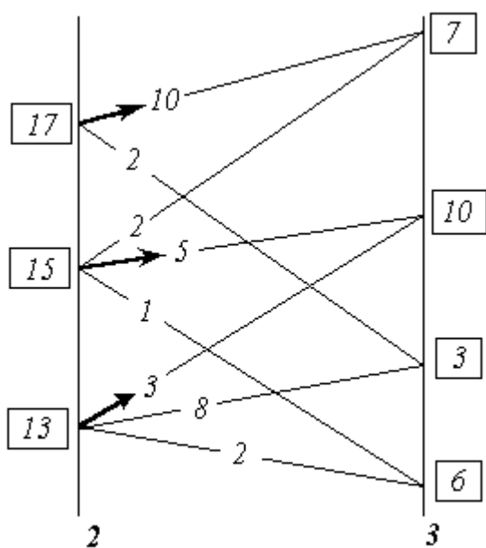
Рис. 2. К существованию метода динамического программирования. Анализ переходов.
