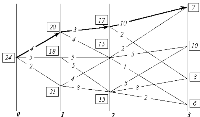
Рис. 3. К СУЩЕСТВУ МЕТОДА ДИНАМИЧЕСКОГО ПРОГРАММИРОВАНИЯ. ОПТИМАЛЬНАЯ ТРАЕКТОРИЯ.
